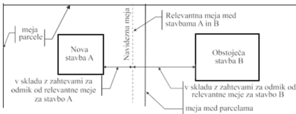
Slika 41: Relevantna in navidezna meja
