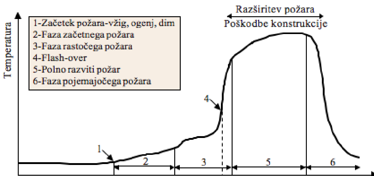
Slika 14: Časovni potek tipičnega požara
