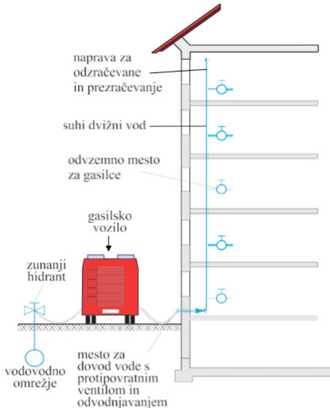
Slika 138: Shematski prikaz suhega dvižnega voda
