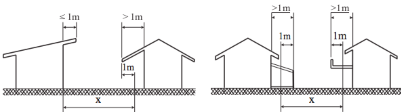
Slika 47: Vpliv nadstreška, balkona ali napušča (VKF)
