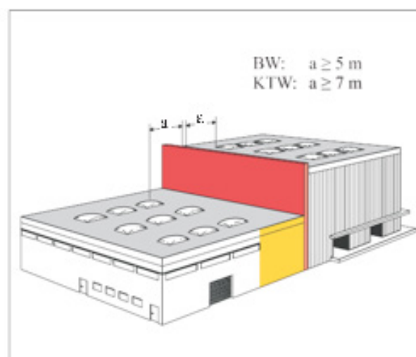
Slika 46: Minimalni zahtevani odmiki med svetlobniki na strehi (VdS 2234)
