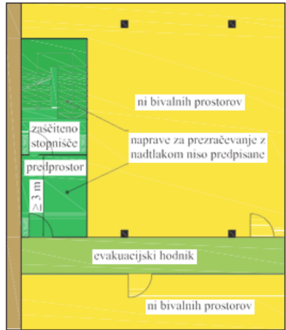
Slika 124: Zahteve za zaščiten stopnišča iz kleti za visoke stavbe po MBO MHHR
