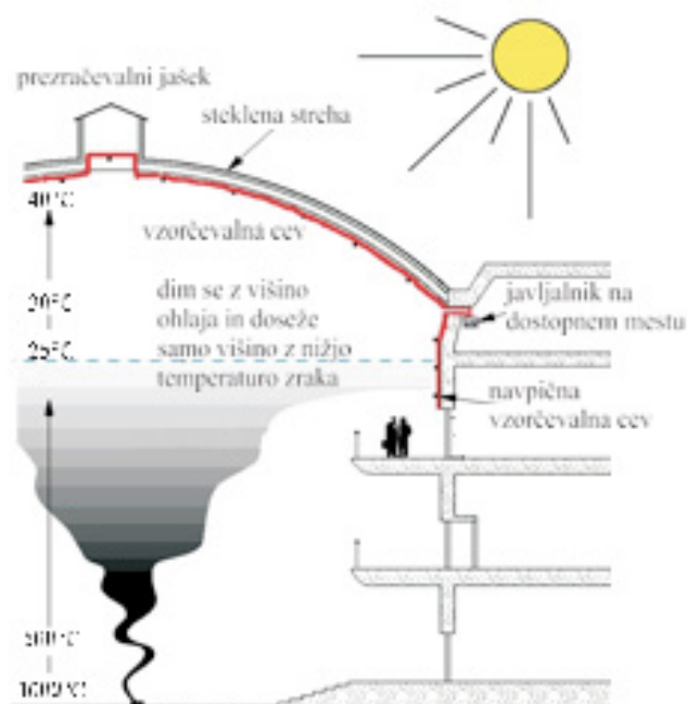
Slika 114: Primer izvedbe sistema javljanja požara v večjih objektih z atrijem
