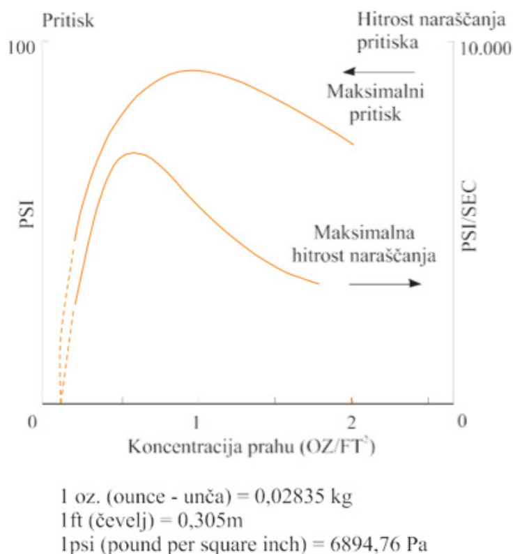
Slika 33: Intenzivnost prašne eksplozije je odvisna od koncentracije prašnih delcev
