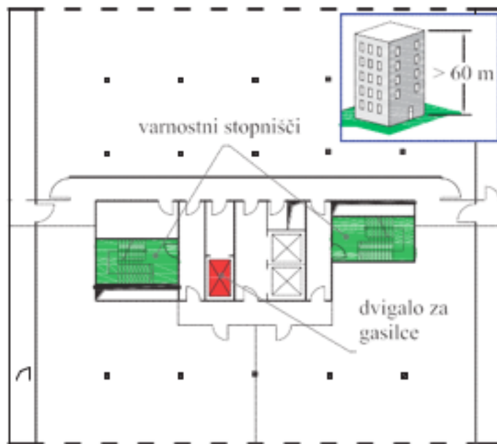
Slika 121: Primer zahtev za evakuacijo za visoke stavbe > 60 m po MBO MHHR
