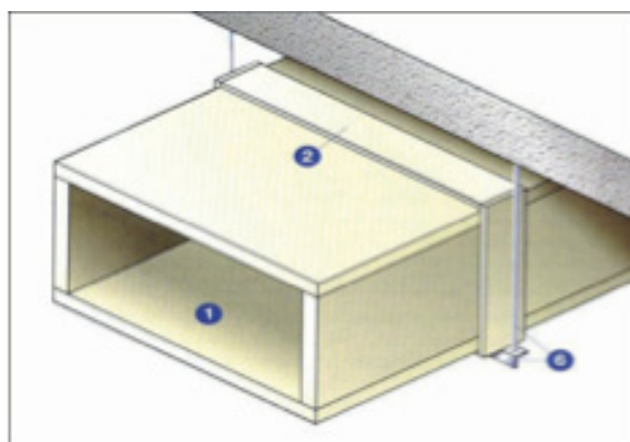
Slika 69: Klasični primer izvedbe MODT v garažah (požarni kanali za ODT)
