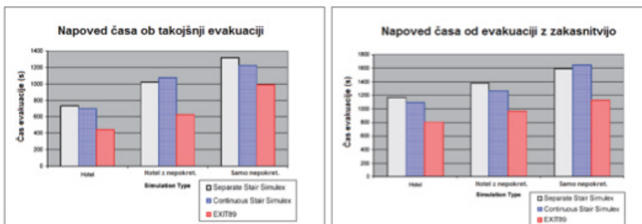
Slika 110: Izračun časov evakuacije
