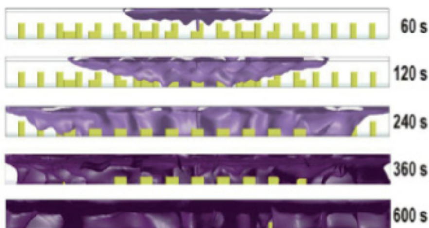
Slika 90: Prečni prerez s slike 89 kaže na razvoj dima in delovanje sistema NODT
