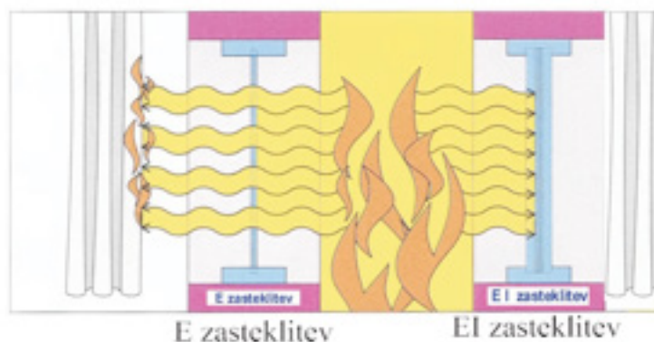
Slika 76: Razlika med E in EI zasteklitvijo
