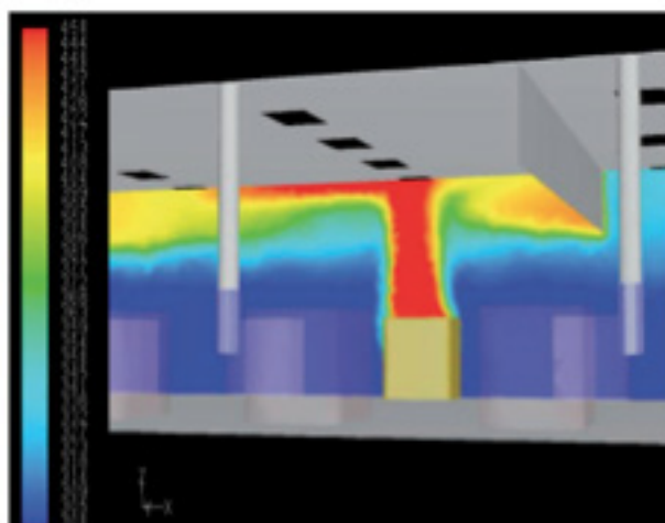
Slika 130: Prostorski prikaz izračunane temperature v simuliranem požaru
