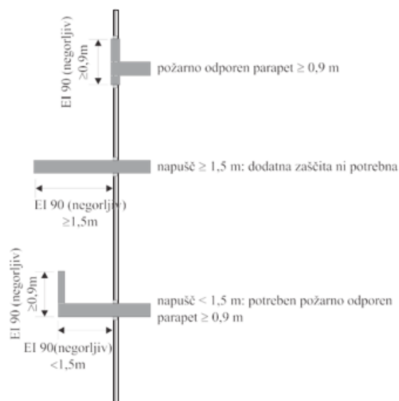
Slika 53: Preprečitev prenosa požara v vertikalni smeri za visoke stavbe po VKF
