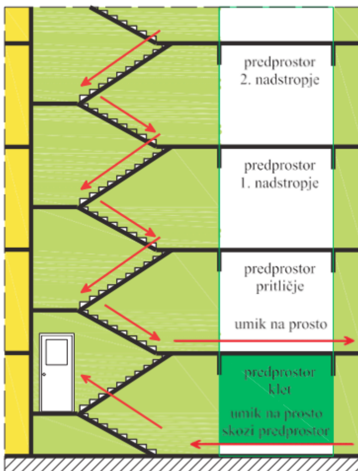
Slika 122: Obvezna ločitev evakuacije iz kleti in nadzemnih etaž za visoke stavbe po MBO MHHR
