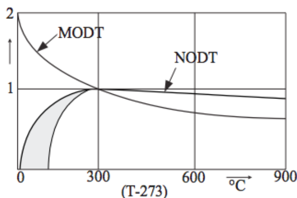
Slika 87: Učinkovitost delovanja NODT in MODT v odvisnosti od temperature dimnih plinov
