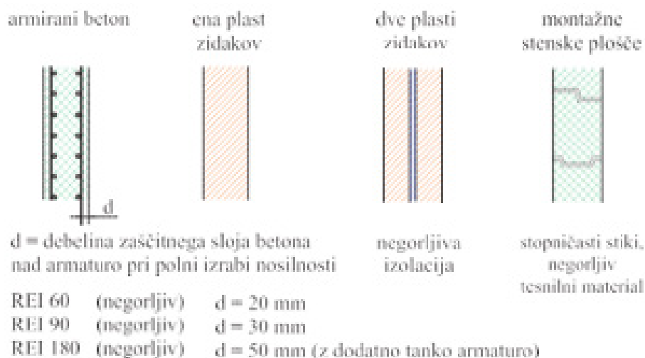
Slika 62: Različne izvedbe zidov za doseg zahtevane požarne odpornosti (VKF)
