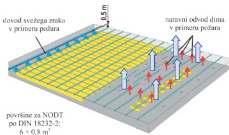
Slika 88: Postavitev sistema NODT: rdeče puščice so odvod dima, modre dovod svežega zraka
