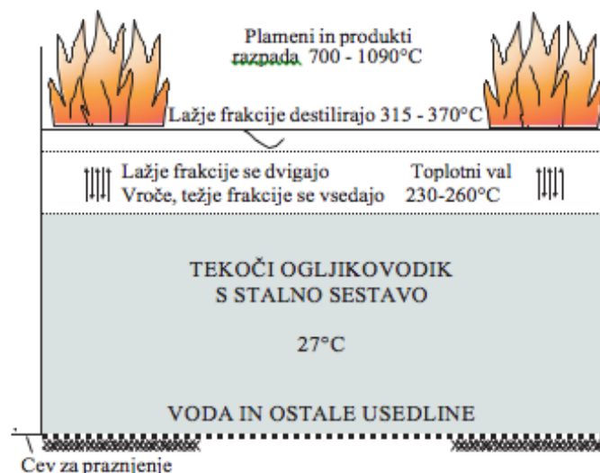
Slika 21: Širjenje toplotnega vala pri požarih težjih naftnih frakcij v rezervoarjih
