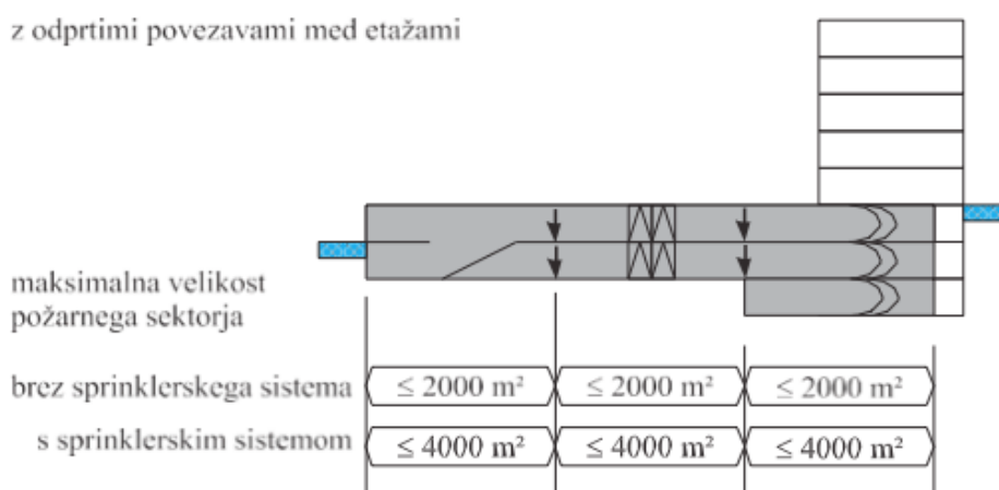
Slika 64: Zahteve za velikosti požarnih sektorjev za stavbo z odprtimi povezavami med etažami (VKF)
