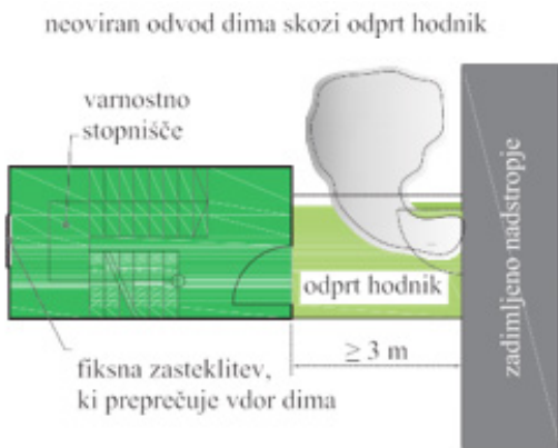
Slika 123: Zahteve za zunanja stopnišča za visoke stavbe po MBO MHHR
