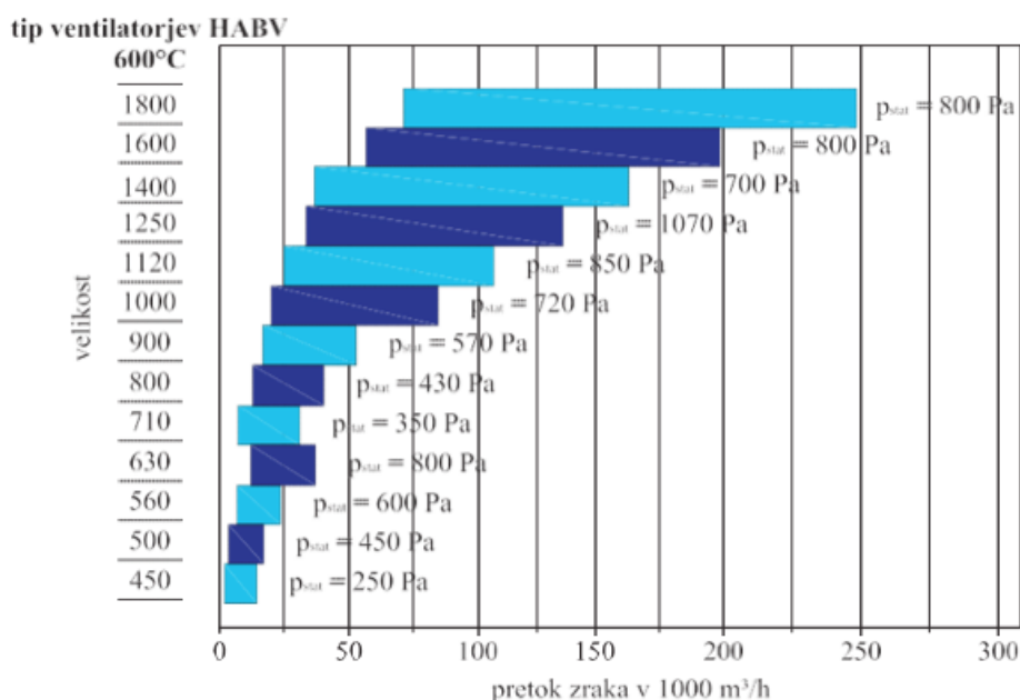
Slika 80: Ventilatorji za MODT (pretoki zraka tudi do 250000 m 3 /h)
