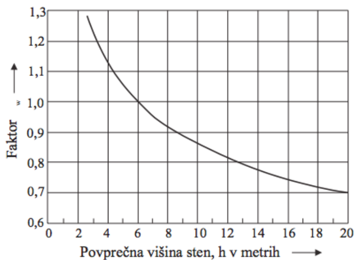
Diagram 4: Faktor \alpha_w (diagram 2, DIN 18230-1)
