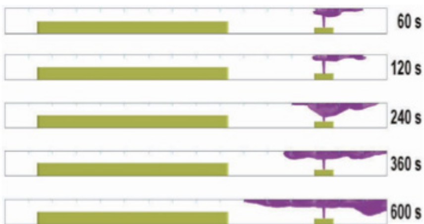
Slika 96: Vzdolžni prerez s slike 94 kaže na razvoj dima in delovanje sistema MODT
