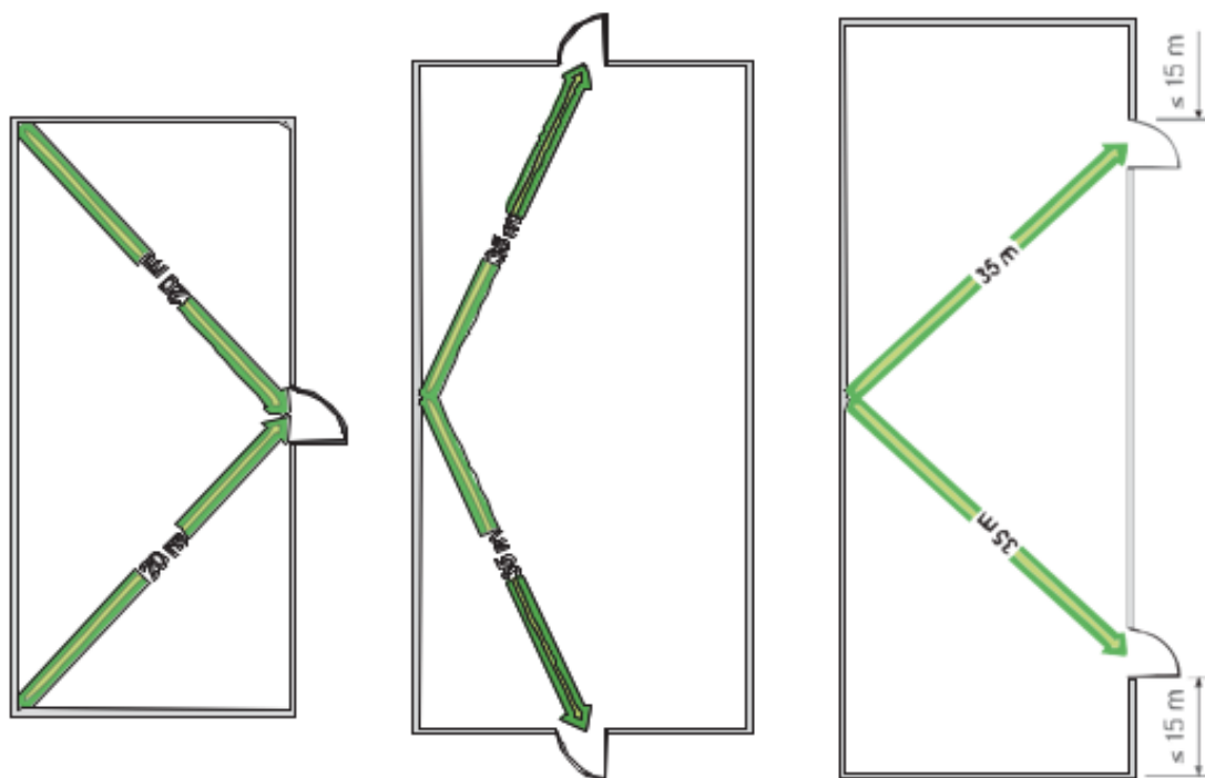
Slika 115: Shematska predstavitev zahtev za izvedbo dolžin evakuacijskih poti glede na število izhodov (VKF)
