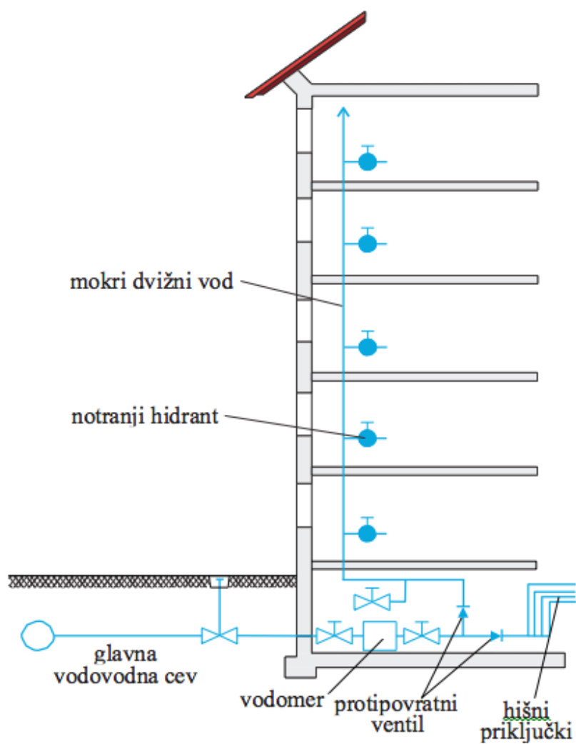
Slika 134: Shematski prikaz mokrega dvižnega voda
