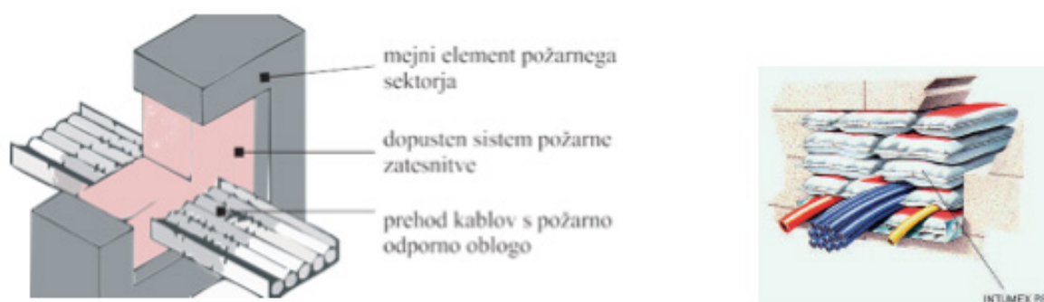
Slika 73: Prehod električnih kablov skozi požarno steno
