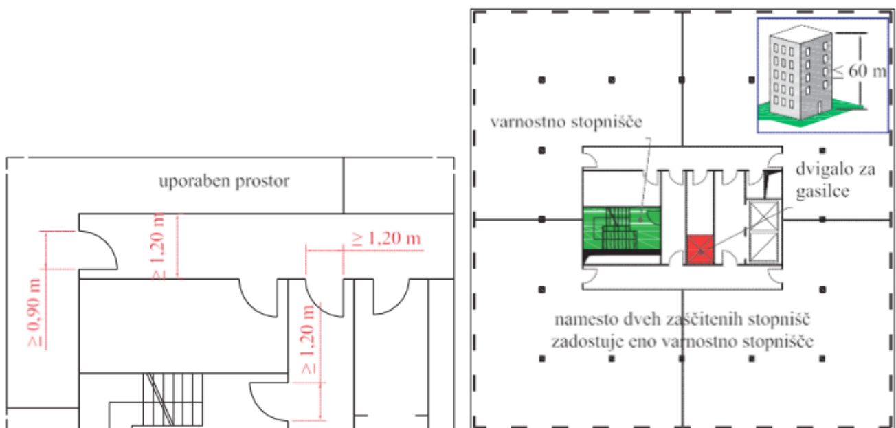
Slika 120: Primer zahtev za evakuacijo za visoke stavbe < 60\text{ m} po MBO MHHR
