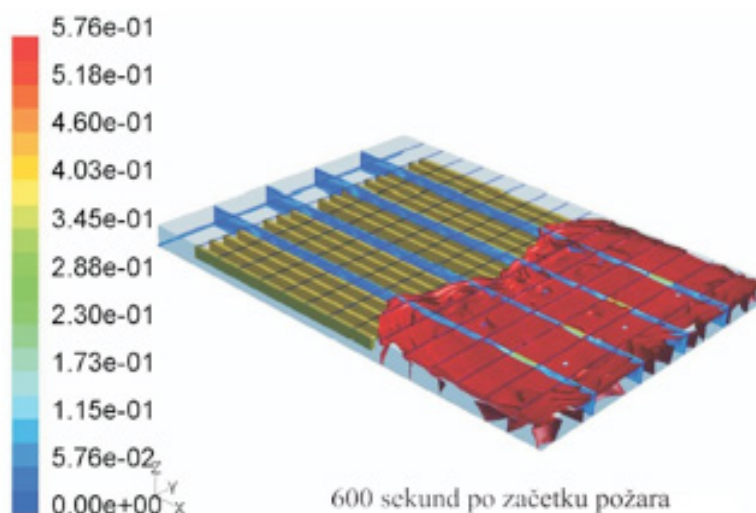
Slika 93: Dim se po 600 s (10 min) širi po vsem prostoru
