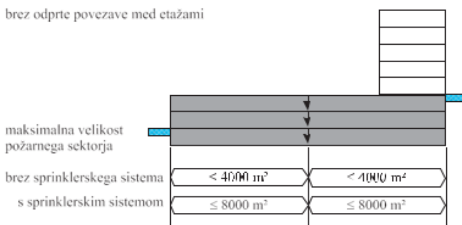
Slika 63: Zahteve za velikosti požarnih sektorjev za stavbo brez odprte povezave med etažami (VKF)
