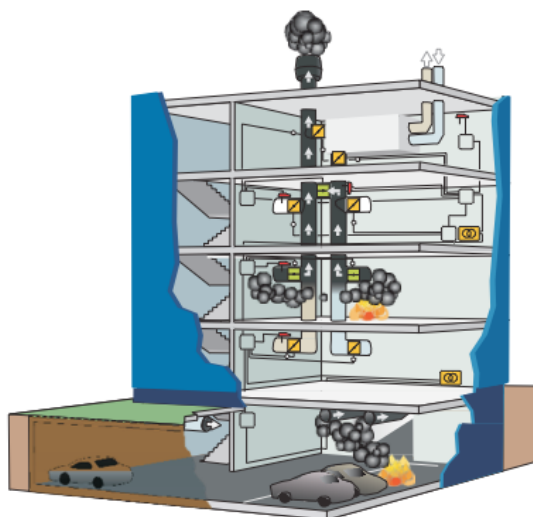
Slika 68: Primer delovanja MODT (mehanskega odvoda dima in toplote) v primeru požara v kleti ali nadstropju
