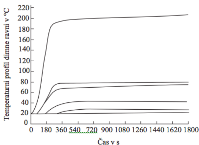
Slika 112: Temperatura dimne ravni v odvisnosti od časa
