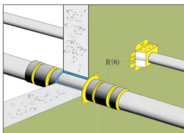
Slika 75: Prehodi skozi meje požarnega sektorja za gorljive cevi (VdS)
