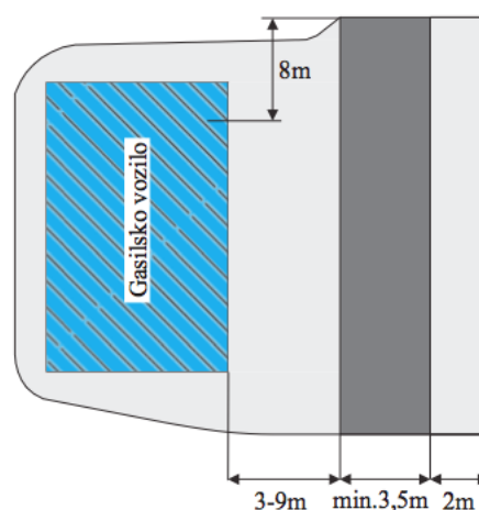
Slika 127: Elementi dostopnih poti in postavitvenih površin
