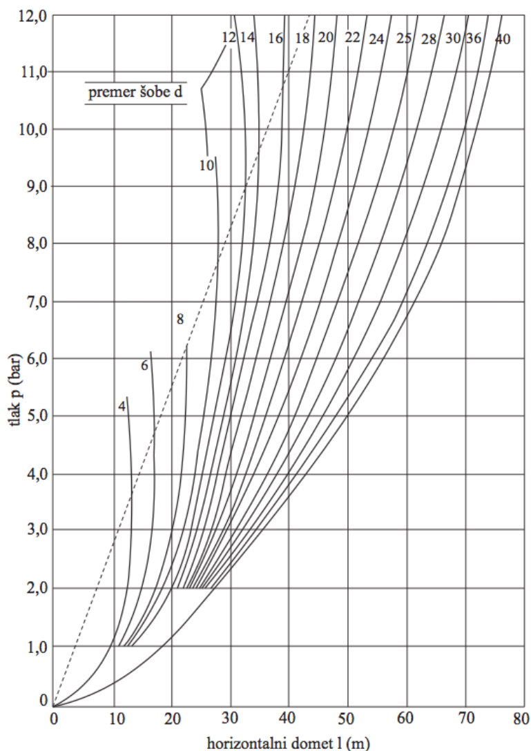
Diagram 6: Največji doomet (m) curka vode v odvisnosti od premera šobe in tlaka na ročniku pri kotu 32°
