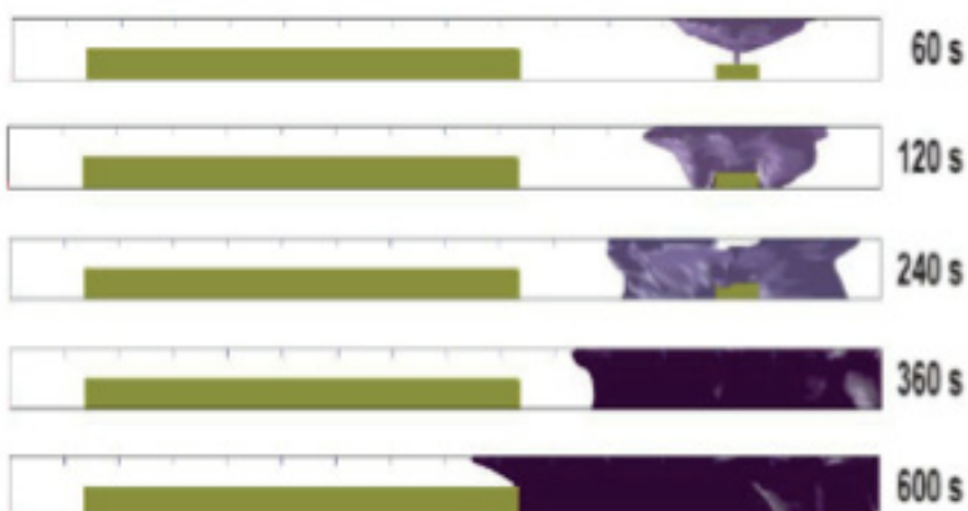
Slika 91: Vzdolžni prerez s slike 89 kaže na razvoj dima in delovanje sistema NODT
