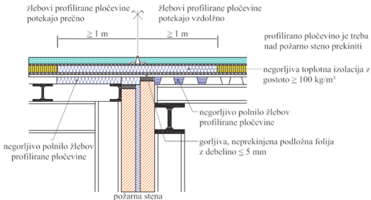
Slika 56: Horizontalna požarna ločitev brez nadvišanja požarnega zidu preko strehe
