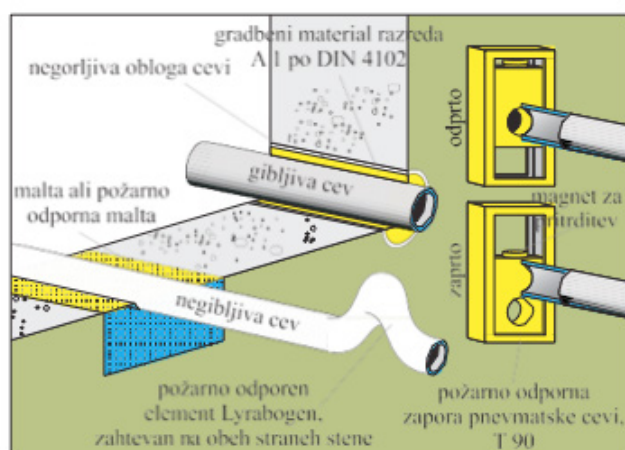
Slika 74: Prehodi skozi meje požarnega sektorja za negorljive cevi (VdS)
