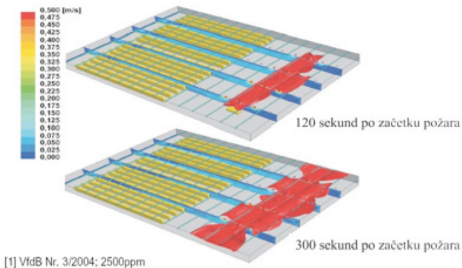
Slika 97: Prikaz zadimljenja z računalniško simulacijo in hitrostni profil
