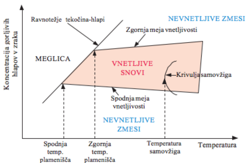
Slika 20: Področje vnetljivosti
