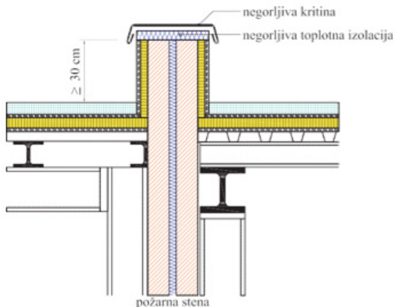
Slika 55: Horizontalna požarna ločitev
