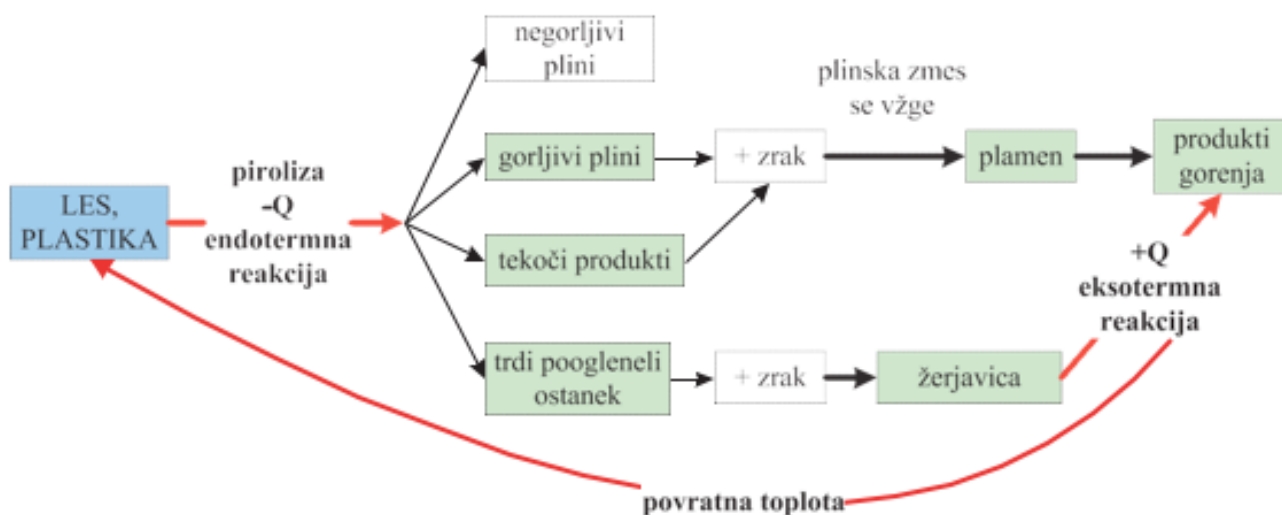
Slika 23: Proces gorenja lesa in plastike
