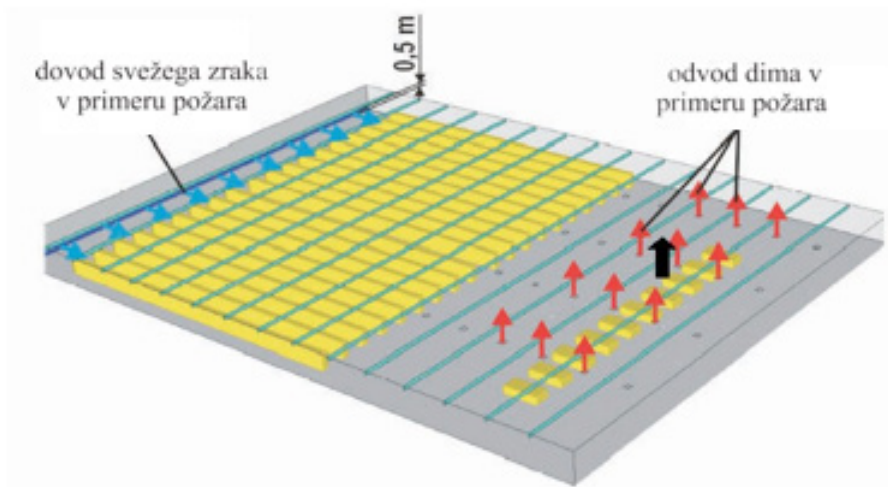
Slika 94: Postavitev sistema MODT: rdeče puščice so odvod dima, modre dovod svežega zraka
