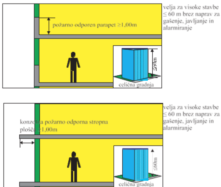
Slika 54: Preprečitev prenosa požara v vertikalni smeri za visoke stavbe po MBO MHHR
