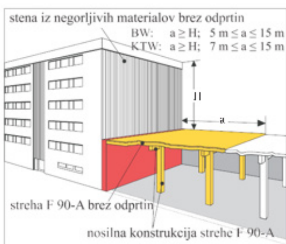
Slika 45: Izvedba strehe sosednje nižje stavbe (VdS 2234)
