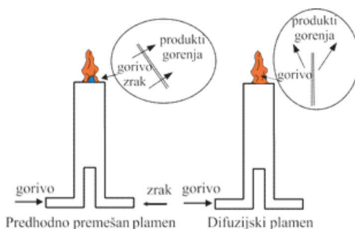
Slika 17: Bunsenov gorilnik – prikaz principa gorenja
