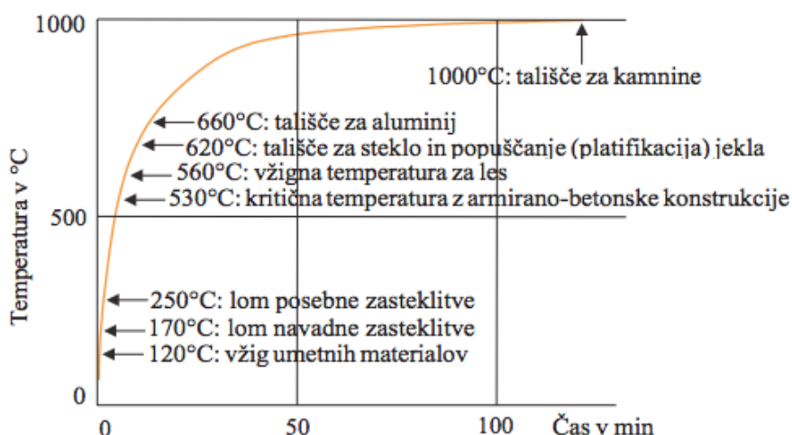
Slika 83: Potek temperature v požaru in vpliv na nosilno konstrukcijo
