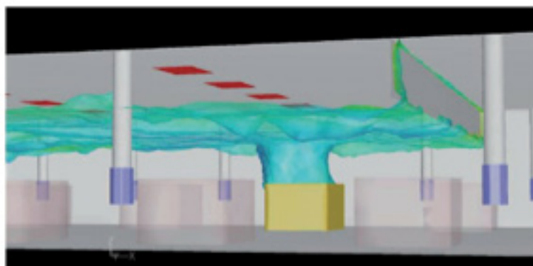
Slika 129: Primer računalniške simulacije požara in širjenja dima po prostoru
