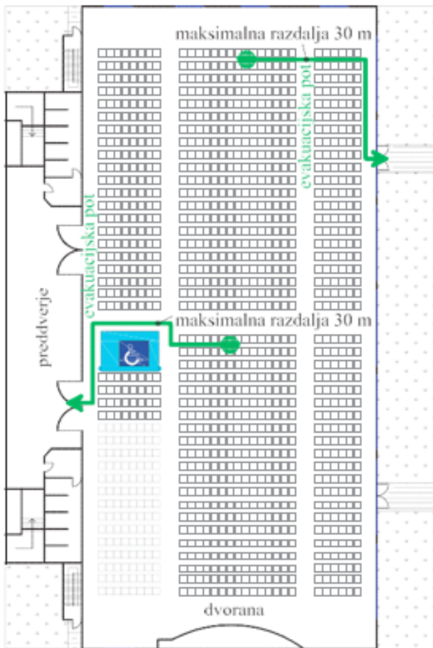
Slika 125: Zahteve za evakuacijo za zbirališča MBO MVStättV
