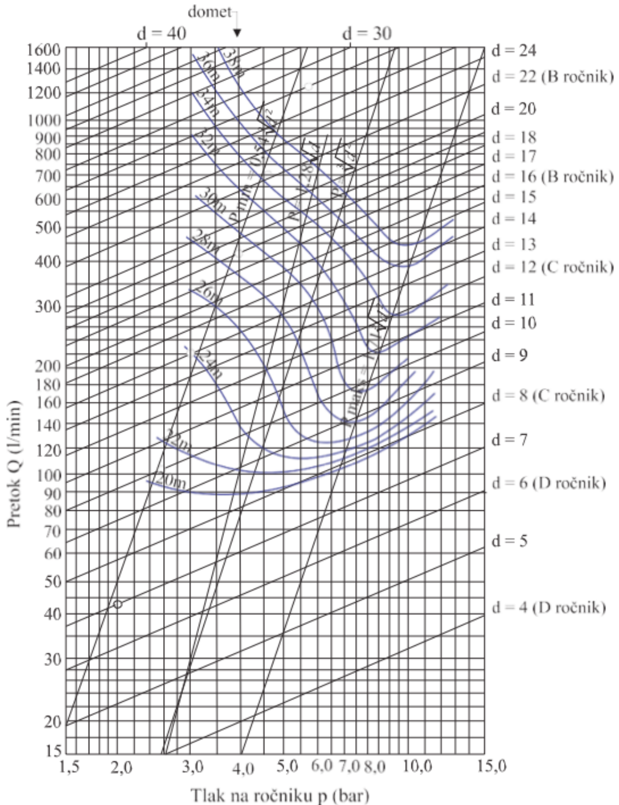
Diagram 5: Pretok vode (l/min) v odvisnosti od tlaka na ročniku in premera šobe
