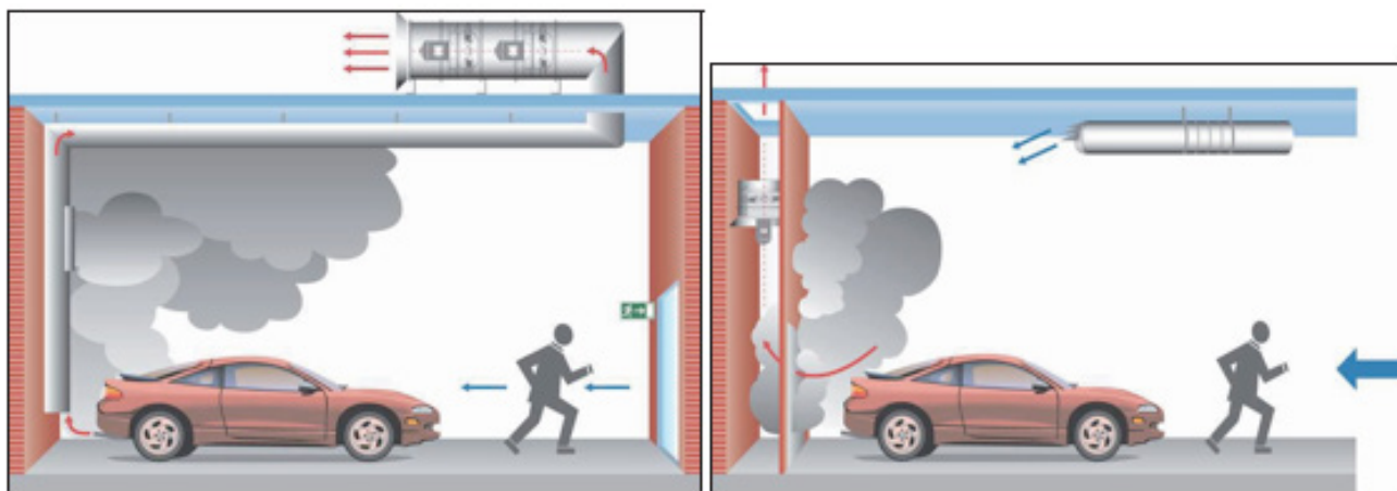
Slika 85: Princip klasičnega sistema odvoda dima in toplote iz garaž – sistem MODT
