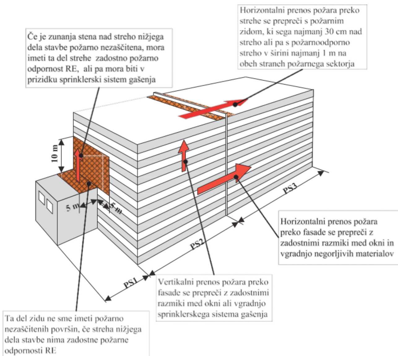
Slika 48: Prenos požara preko zunanjih sten in strehe
