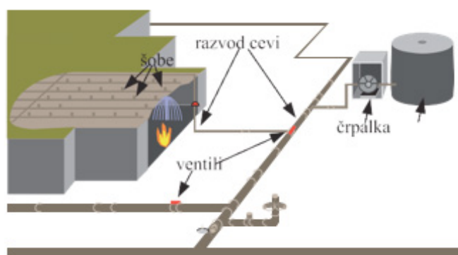
Slika 103: Shematski prikaz sprinklerske instalacije
