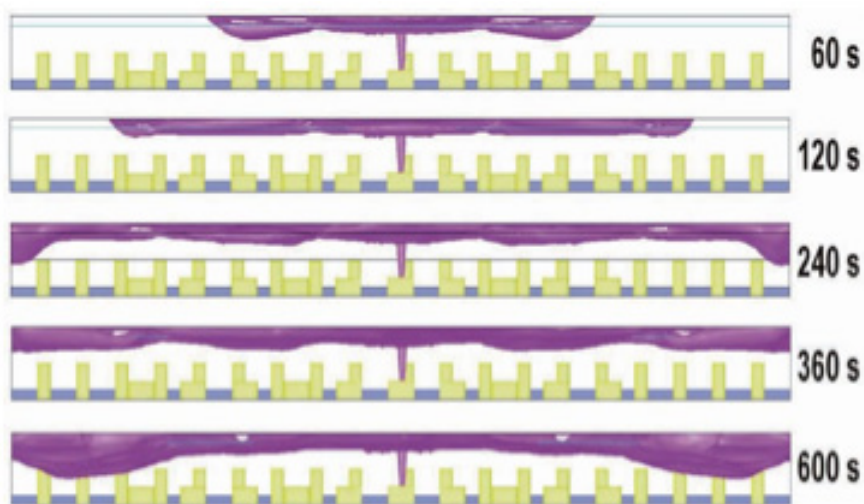
Slika 95: Prečni prerez s slike 94 kaže na razvoj dima in delovanje sistema MODT
