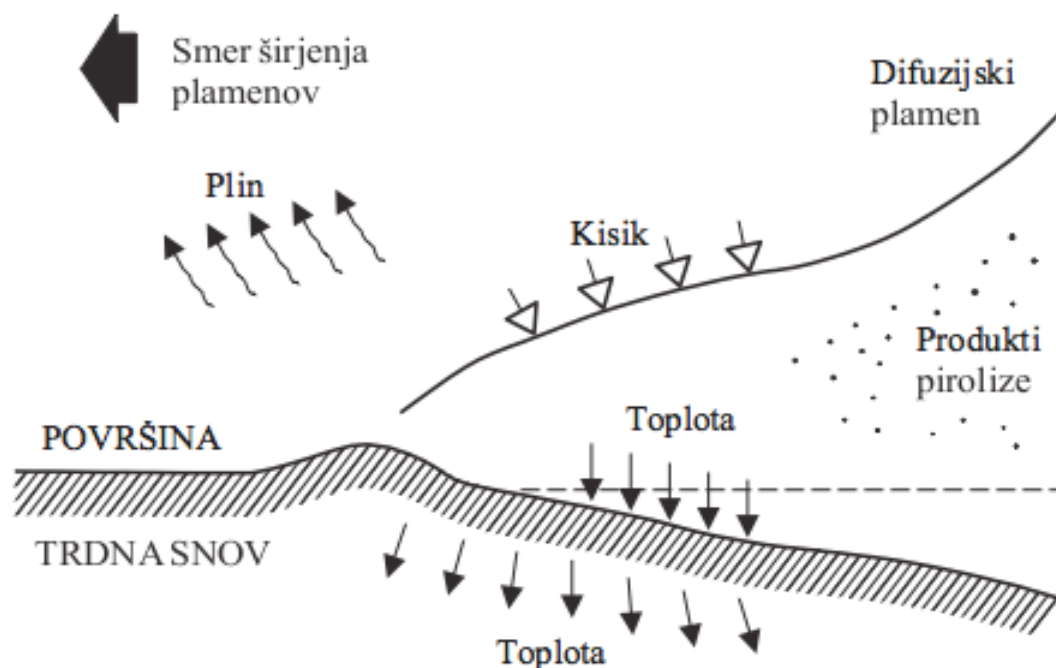
Slika 25: Širjenje plamenov pri gorenju trdnih materialov
