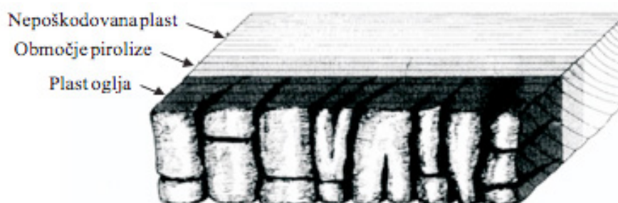
Slika 24: Proces pirolize
