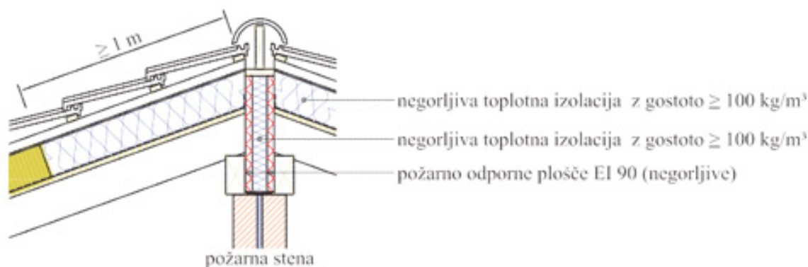
Slika 57: Horizontalna požarna ločitev preko slemena
