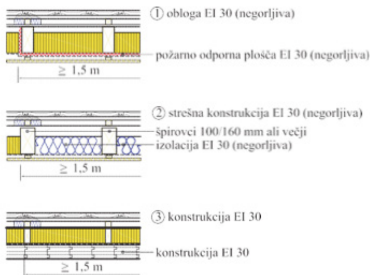
Slika 50: Primeri detajlov požarne zaščite na stikih iz slike 49 (VKF)
