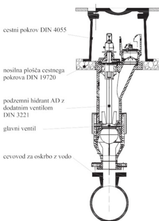
Slika 132: Direktna priključitev na cevovod – podzemni hidrant (po DIN 3221-1)
