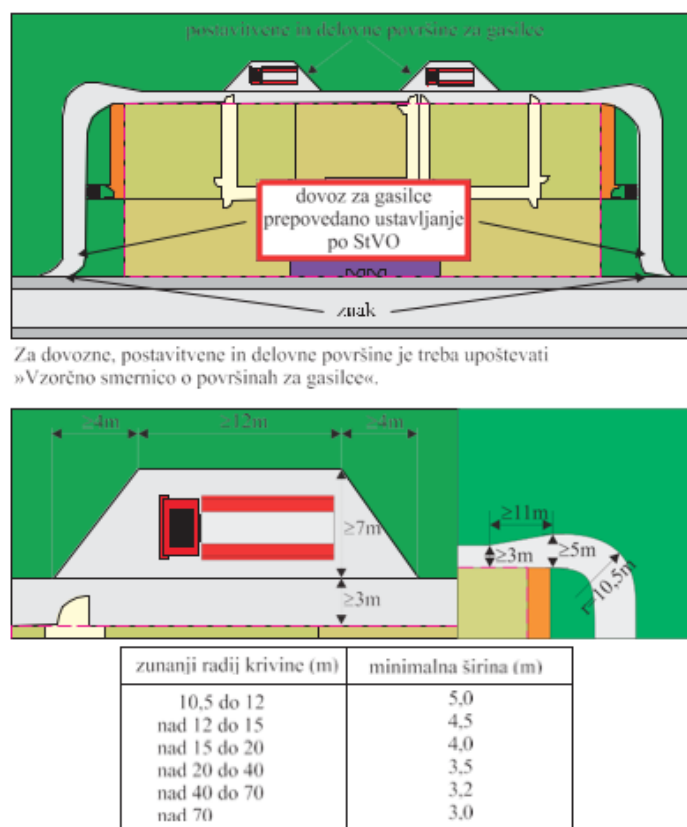
Slika 5: Primer postavitvenih in dovoznih poti za gasilce po nemškem MBO MHHR
