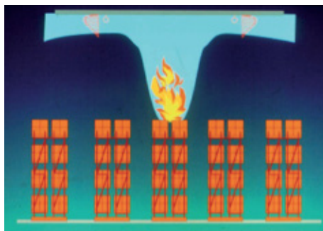
Slika 109: Sproščanje dima in toplote pri požaru v regalnem skladišču proži sprinklerje
