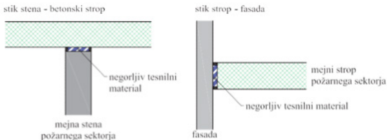
Slika 61: Detajli spojev med zunanjo steno in notranjo steno med požarnimi sektorji (VKF)
