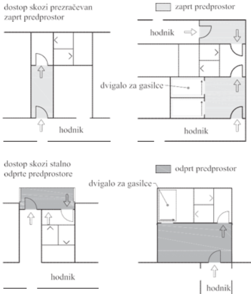
Slika 119: Primer zahtev za predprostore za visoke stavbe (VKF)
