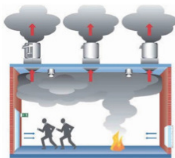
Slika 82: Shematski prikaz mehanskega odvoda dima
