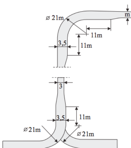
Slika 126: Elementi dostopnih poti in postavitvenih površin
