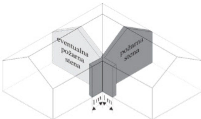
Slika 59: Preprečen prenos požara preko notranjega vogala
