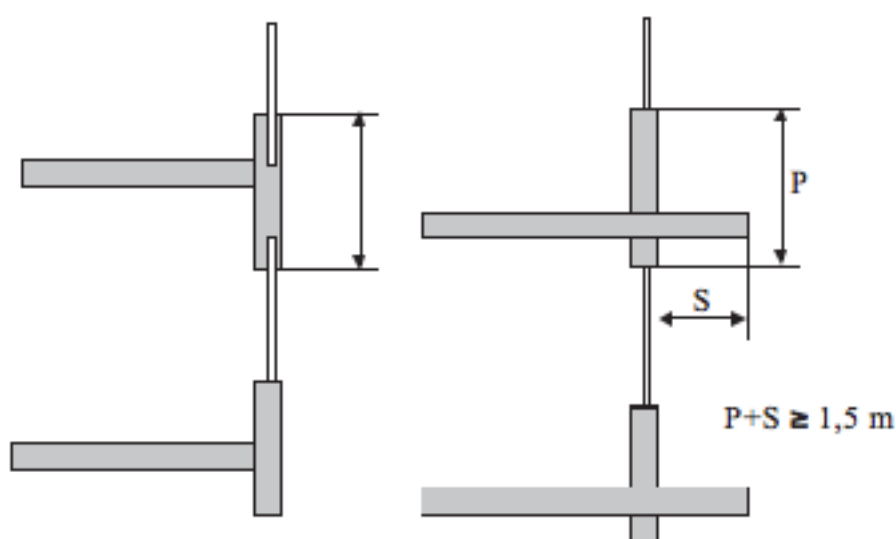
Slika 52: Vertikalni razmik med okni v zunanji steni visokih stavb
