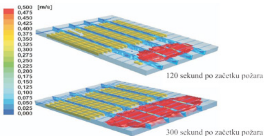
Slika 92: Prikaz zadimljenja z računalniško simulacijo in hitrostni profil, v času 120 s in 300 s
