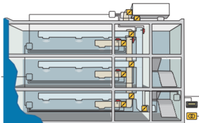
Slika 67: Shematski prikaz MODT (mehanskega odvoda dima in toplote) po etažah in s stopnišča
