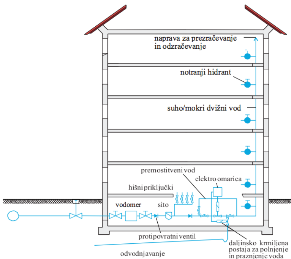
Slika 135: Shematski prikaz suho/mokrega dvižnega voda
