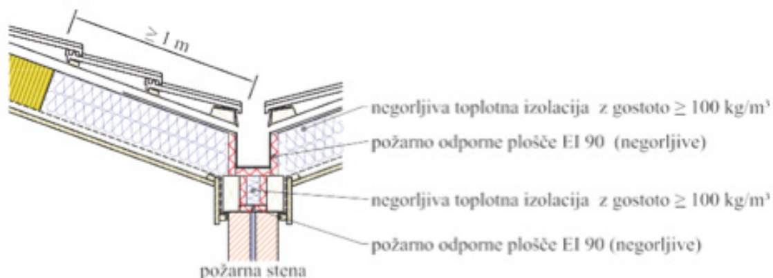
Slika 58: Horizontalna požarna ločitev preko žleba
