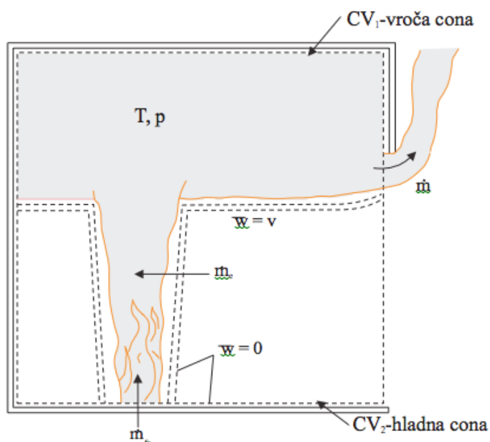
Slika 128: Razdelitev prostora na dve coni
