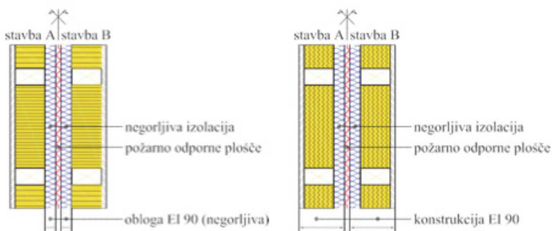
Slika 51: Požarna stena montažne lesene izvedbe, VdS
