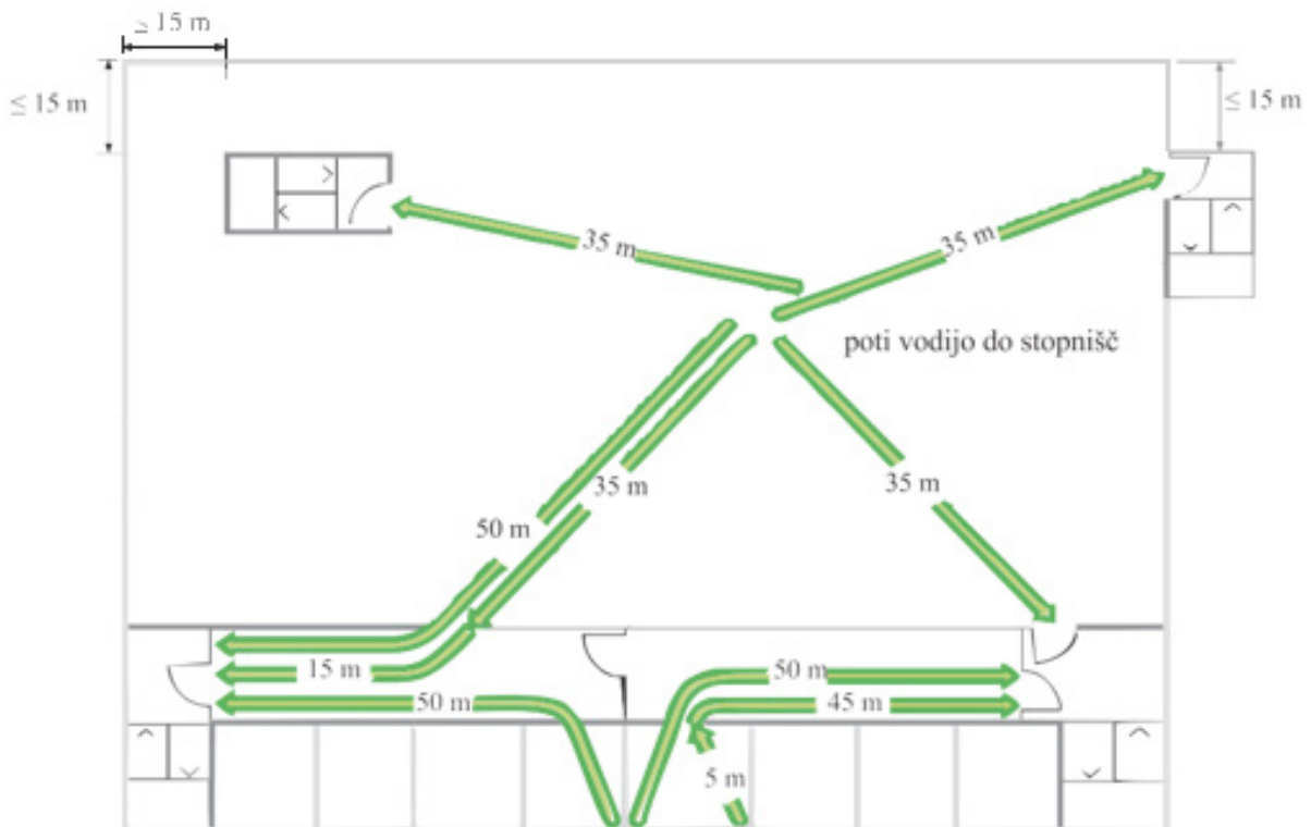
Slika 118: Primer zahtev za evakuacijo z več stopnišči (VKF)
