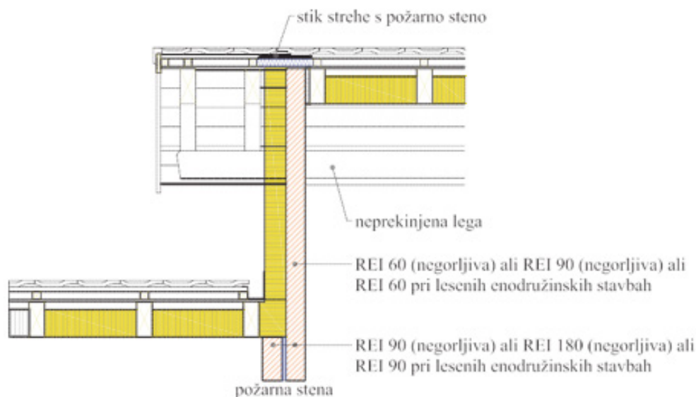
Slika 49: Primer detajla požarne zaščite na stiku višje in nižje stavbe, VKF
