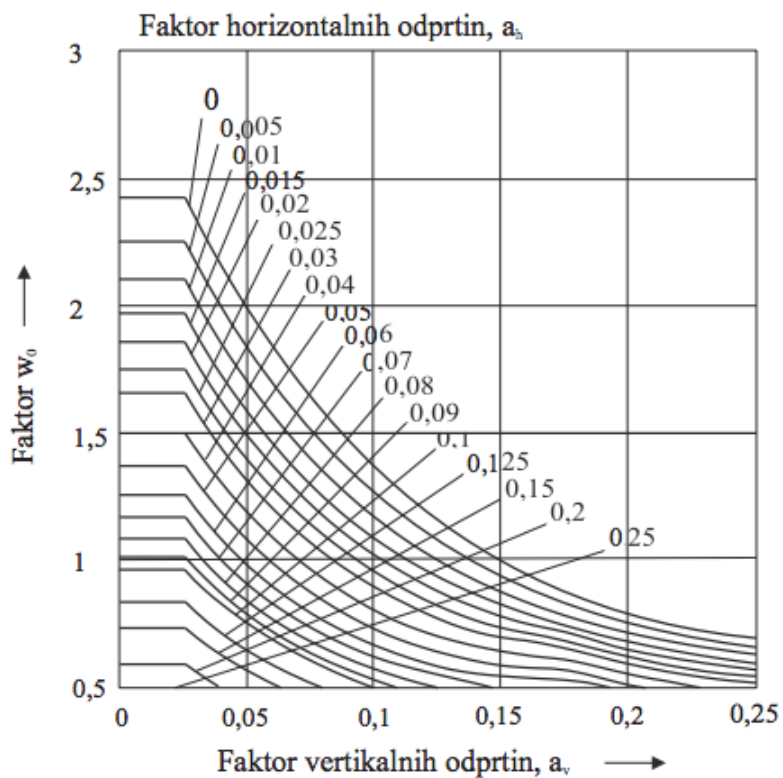
Diagram 4: Faktor \alpha_w (diagram 2, DIN 18230-1)
