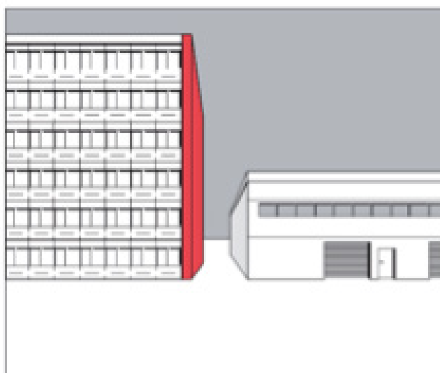
Slika 43: Požarna stena med stavbama, ko je odmik premajhen (VdS 2234)
