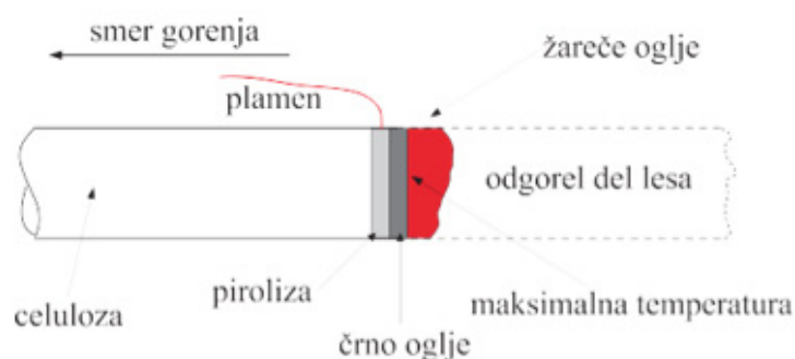
Slika 26: Območje plamena in območje pirolize pri trdnih snoveh
