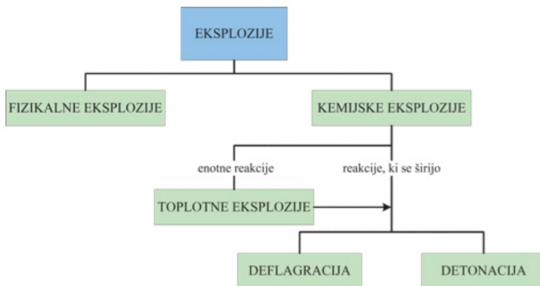
Slika 30: Vrste eksplozij glede na izvor
