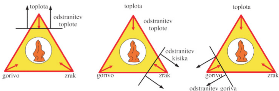
Slika 34: Osnovni mehanizmi gašenja
