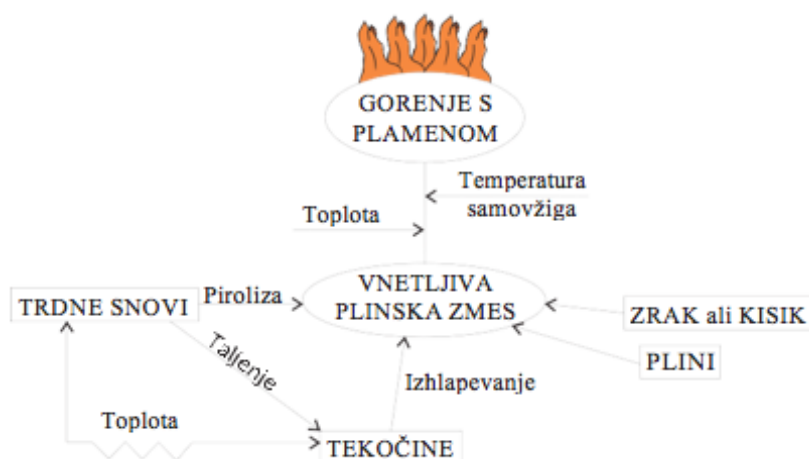
Slika 19: Gorenje s plamenom
