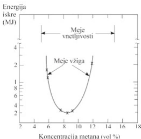
Slika 32: Energija vžiga v odvisnosti od koncentracije
