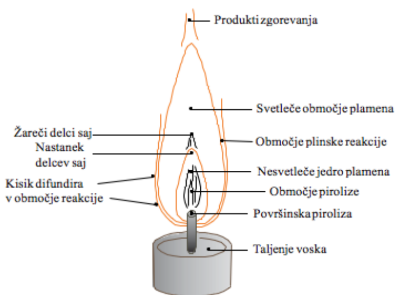
Slika 22: Proces, ki potekajo pri gorenju s taljenjem
