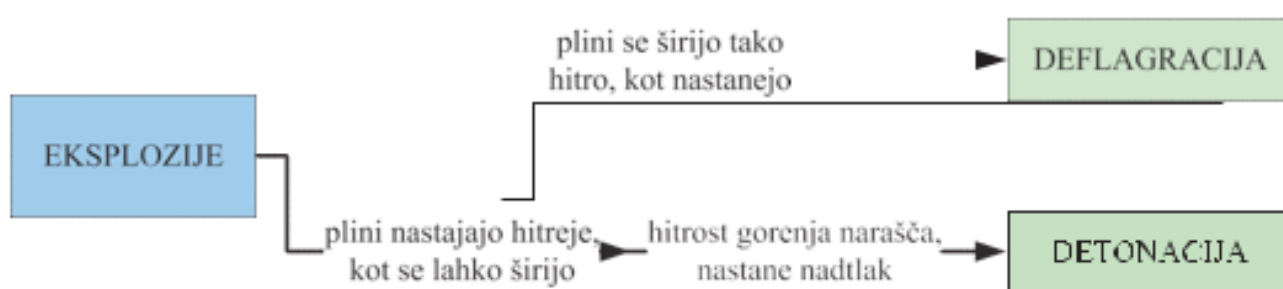
Slika 31: Pogoji, ki določajo nastanek deflagracije in detonacije
