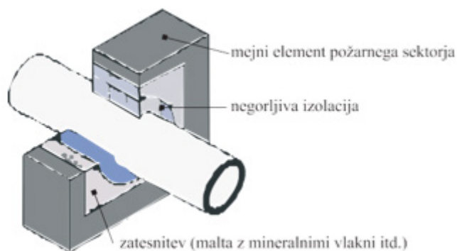
Slika 70: Prehod negorljive cevi skozi požarno steno
